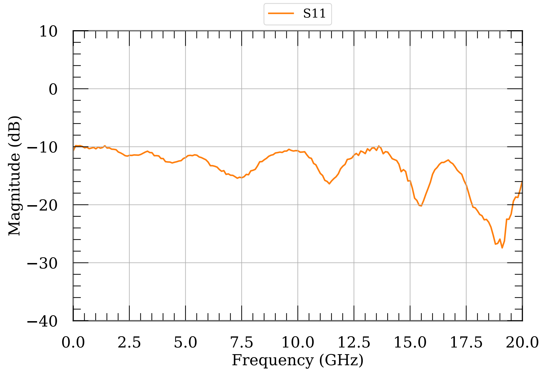
LNA S-params module100
